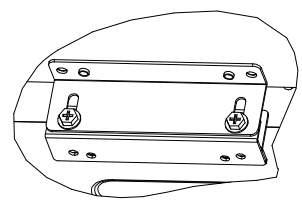
DETAIL B 2:1
